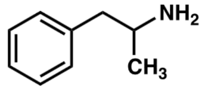
( RS )-1-phenylpropan-2-amine
