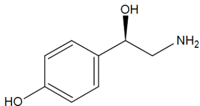
R -(-)-Octopamine
